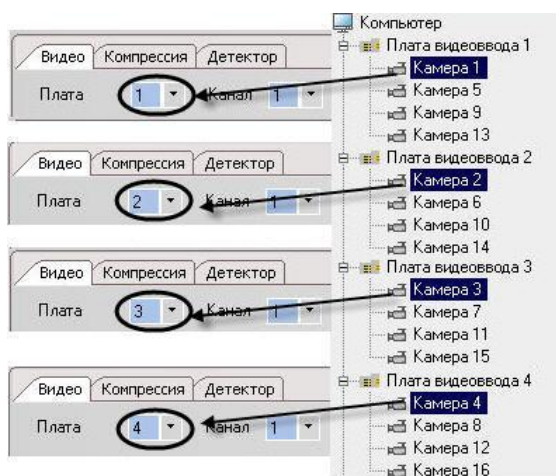
Рис. 5.1-2. Распределение объектов «Камера» на АЦП платы FS4
