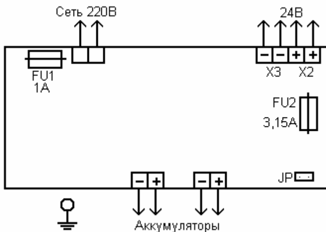
Рис. 1 Схема внешних соединений «ПАРУС-7М»
