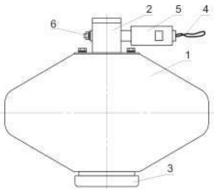
Рис. 1. Конструкция МПП «Гарант-7» во взрывозащищённом исполнении
